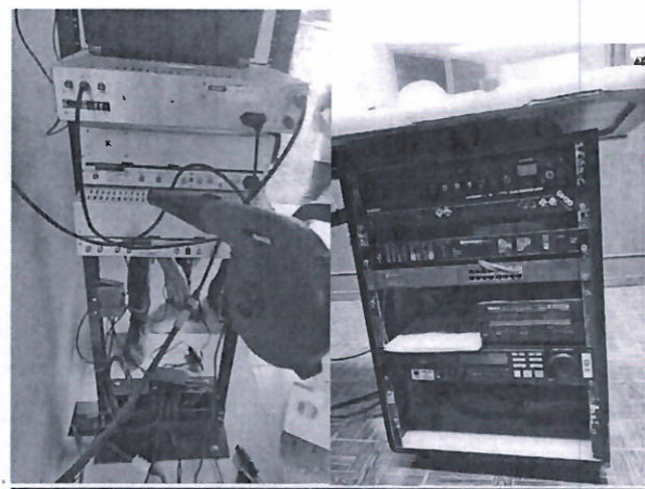
Limpieza de rack de equipos en caseta de transmisión y rack de equipos de audio en cabina de transmisión.
